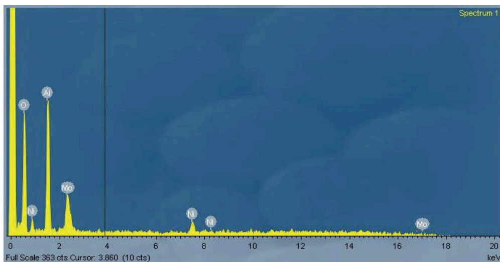
Сурет 5. Ni-Mo-ПЭГ/Al 2 O 3 жүйесінің EDS спектрі.
