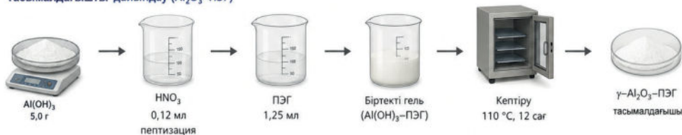
Тасымалдағышты дайындау ( \text{Al}_2\text{O}_3 -ПЭГ)
