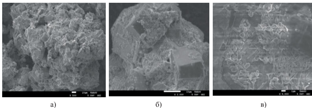
Сурет 3. Әртүрлі ажыратымдылықтағы Со-Мо-ПЭГ/ \text{Al}_2\text{O}_3 СЭМ микрофотографиялары: а – 500; б – 2000; в – 5000.
