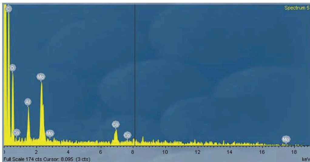
Сурет 4. Co-Mo-ПЭГ/ \text{Al}_2\text{O}_3 жүйесінің EDS спектрі.
