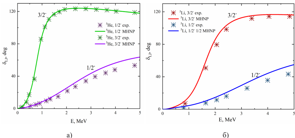
Сурет 3. а) \frac{3}{2}^- және \frac{1}{2}^- кванттық сандарымен алынған {}^5_2\text{He} ядросының б) \frac{3}{2}^- және \frac{1}{2}^- кванттық сандарымен алынған {}^5_3\text{Li} ядросының МННП потенциалын қолдану арқылы AV RGM әдісімен алынған фазалық ығысуларының (δ) шашырау энергиясынан (E) тәуелділігі.
