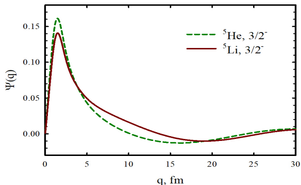
Сурет 2. {}^5\text{He} және {}^5\text{Li} ядроларының негізгі күйлерінің координаталық кеңістіктегі J^\pi = \frac{1}{2}^- толқындық функциялары.
