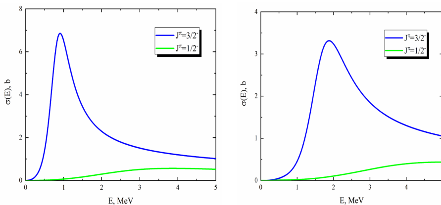
Сурет 1. а) \alpha + {}^1_0n \rightarrow {}^5_2\text{He} реакциясының шашырау қималары. б) \alpha + {}^1_1p \rightarrow {}^5_3\text{Li} реакциясының шашырау қималары.
