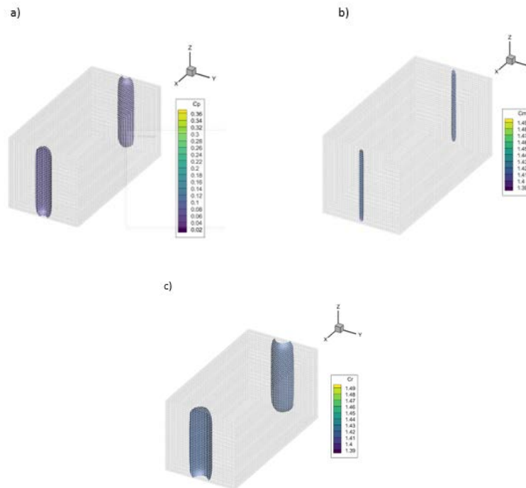
5-сурет. Концентрация таралуының 3D көріністері, t=100 тәулік: а) сұйық фазадағы пайдалы компонент, б) қатты фазадағы пайдалы компонент, с) реагент.
